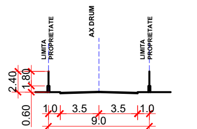
SECTIUNE ARTERA CIRCULATIE
